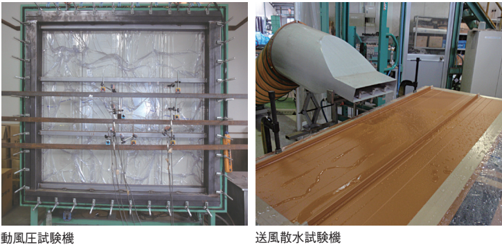
動風圧試験機
